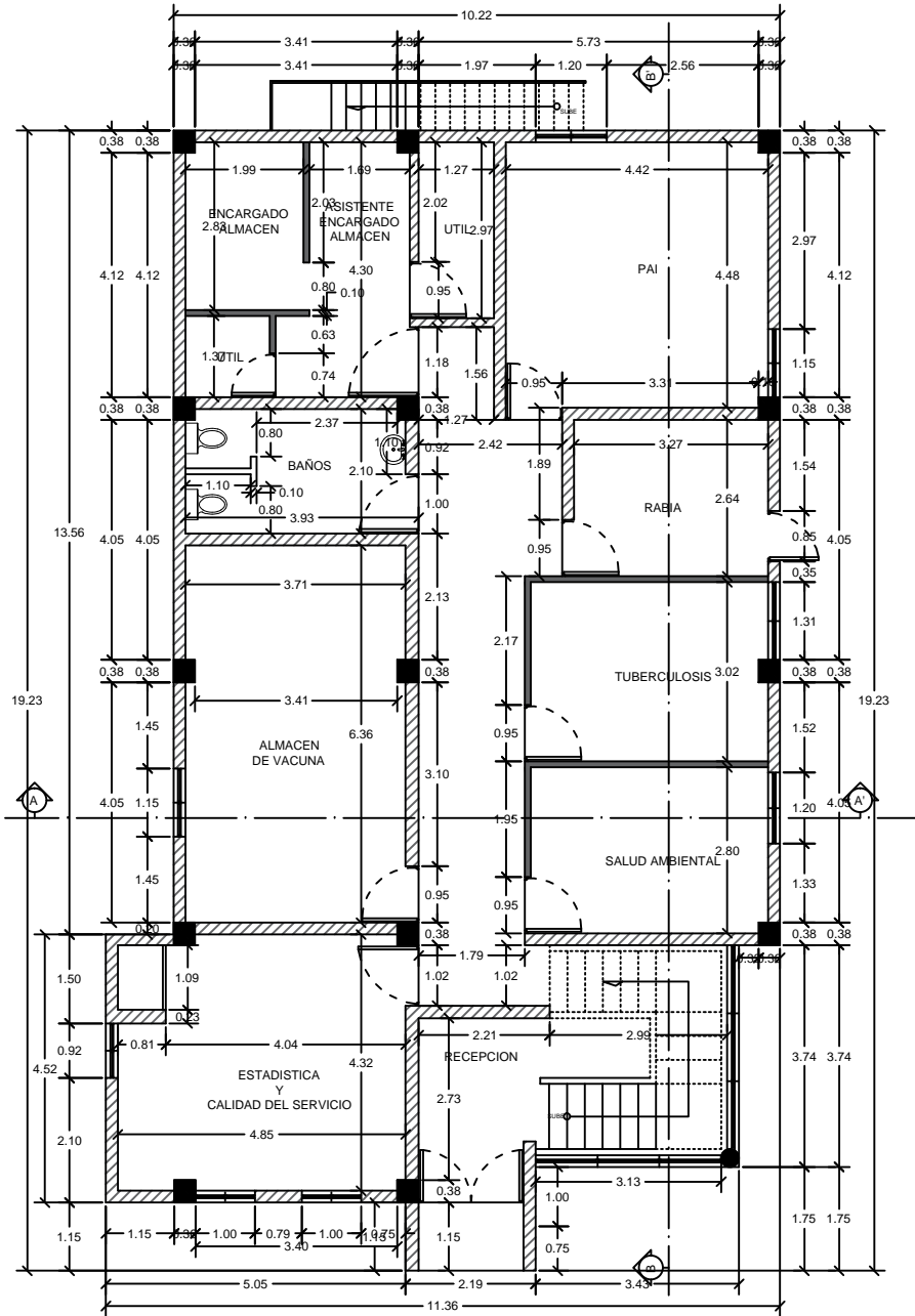
LEVANTAMIENTO DIMENSIONADO ACTUAL 1ER NIVEL
