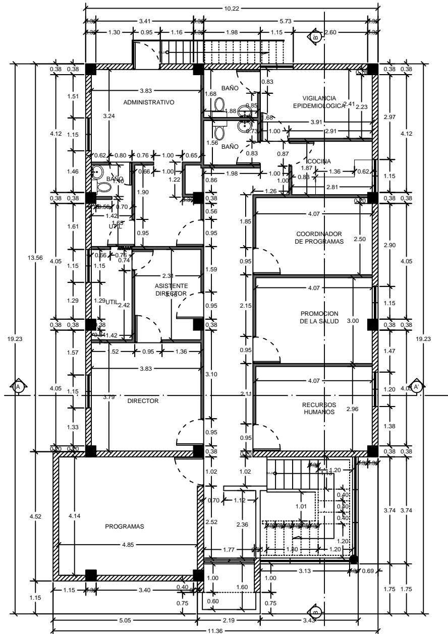
LEVANTAMIENTO DIMENSIONADO ACTUAL 2DO NIVEL
