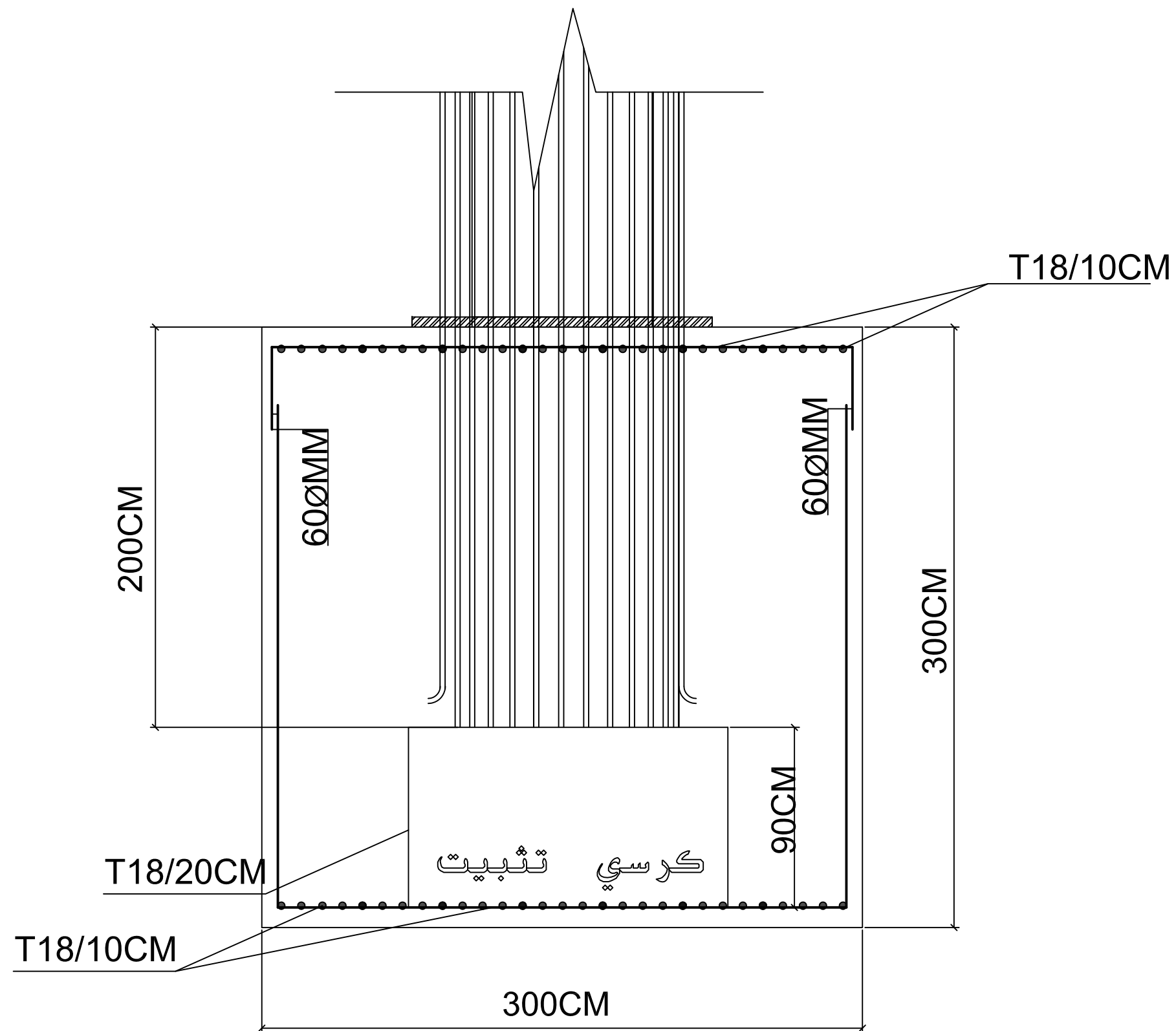
SECTION A-A
