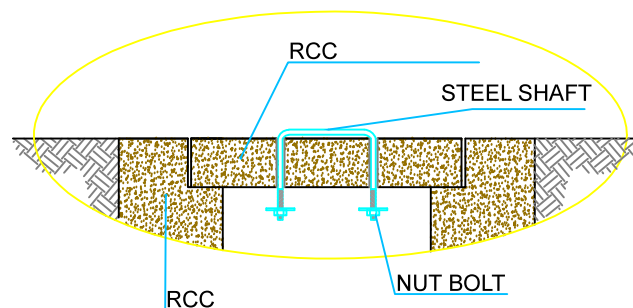
2 E-07 DETAILA Scale:NOT
