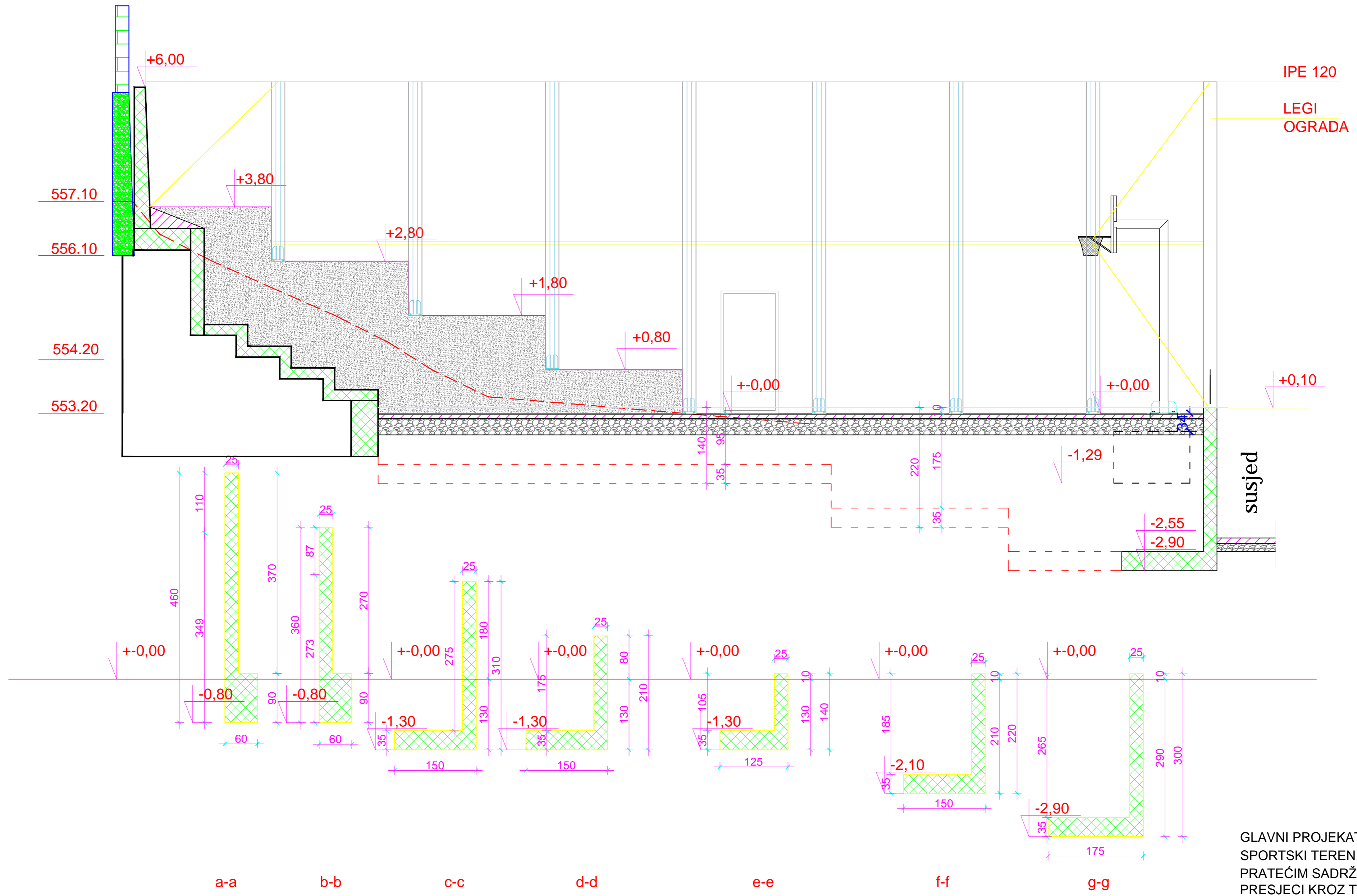
PRESJECI KROZ TEMELJNE ZIDOVE (T.Z.)
