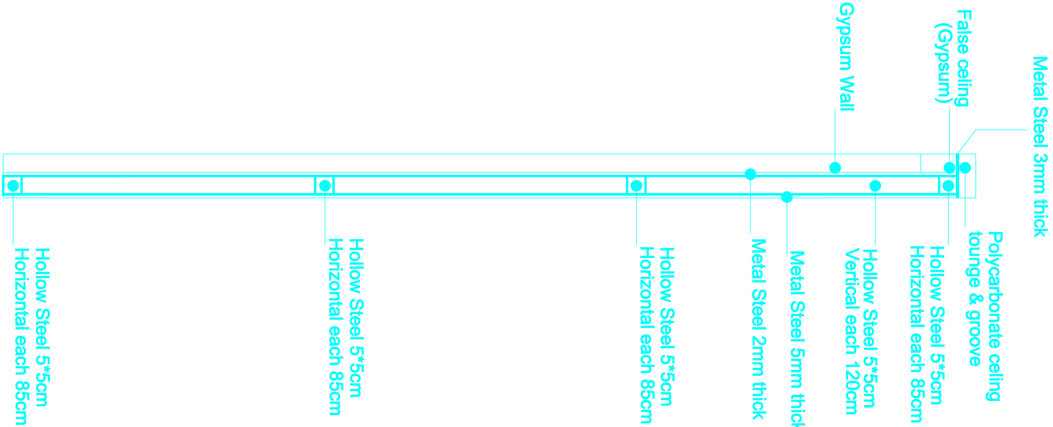
SECTION A-A
