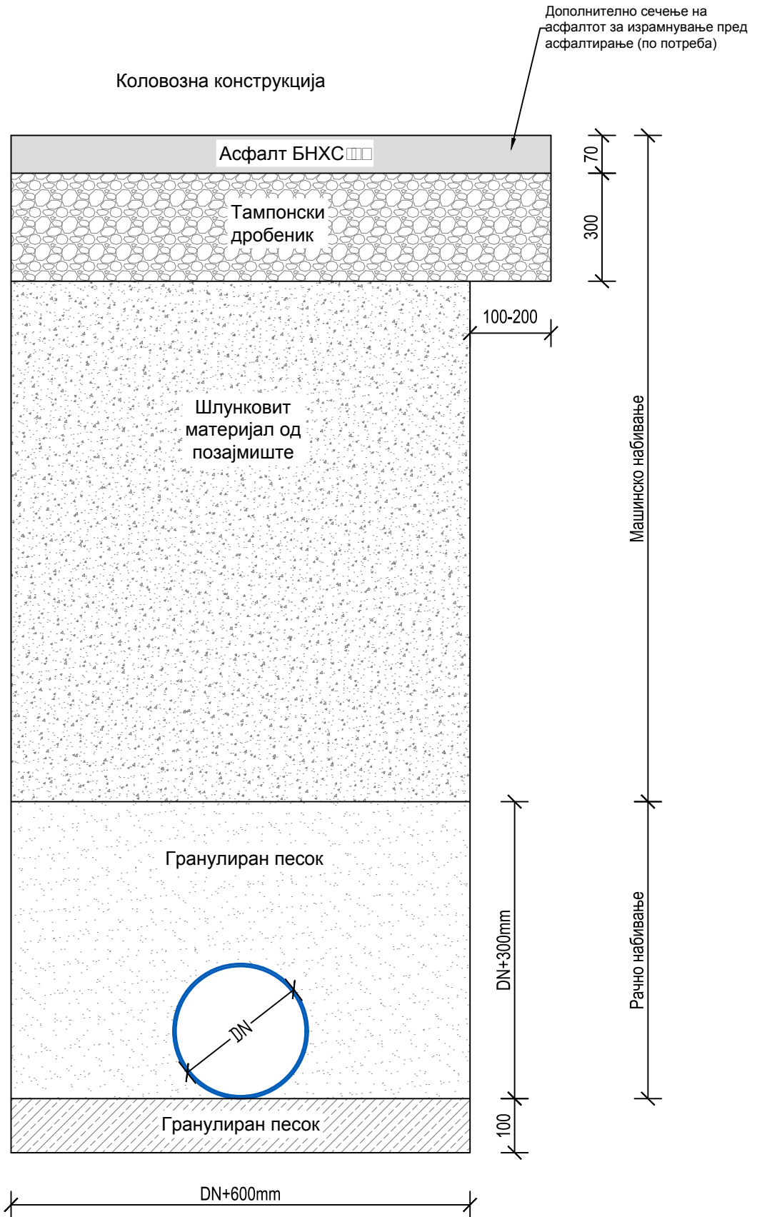
КАРАКТЕРИСТИЧЕН ПОПРЕЧЕН ПРЕСЕК НА РОВ - КОЛОВОЗ
