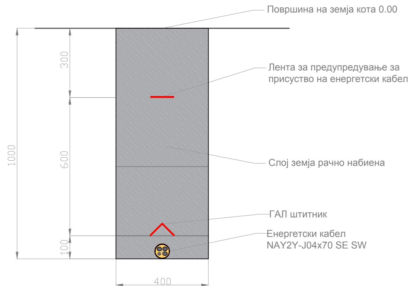
Попречен пресек на ров за водење на енергетски кабел M=1:10
