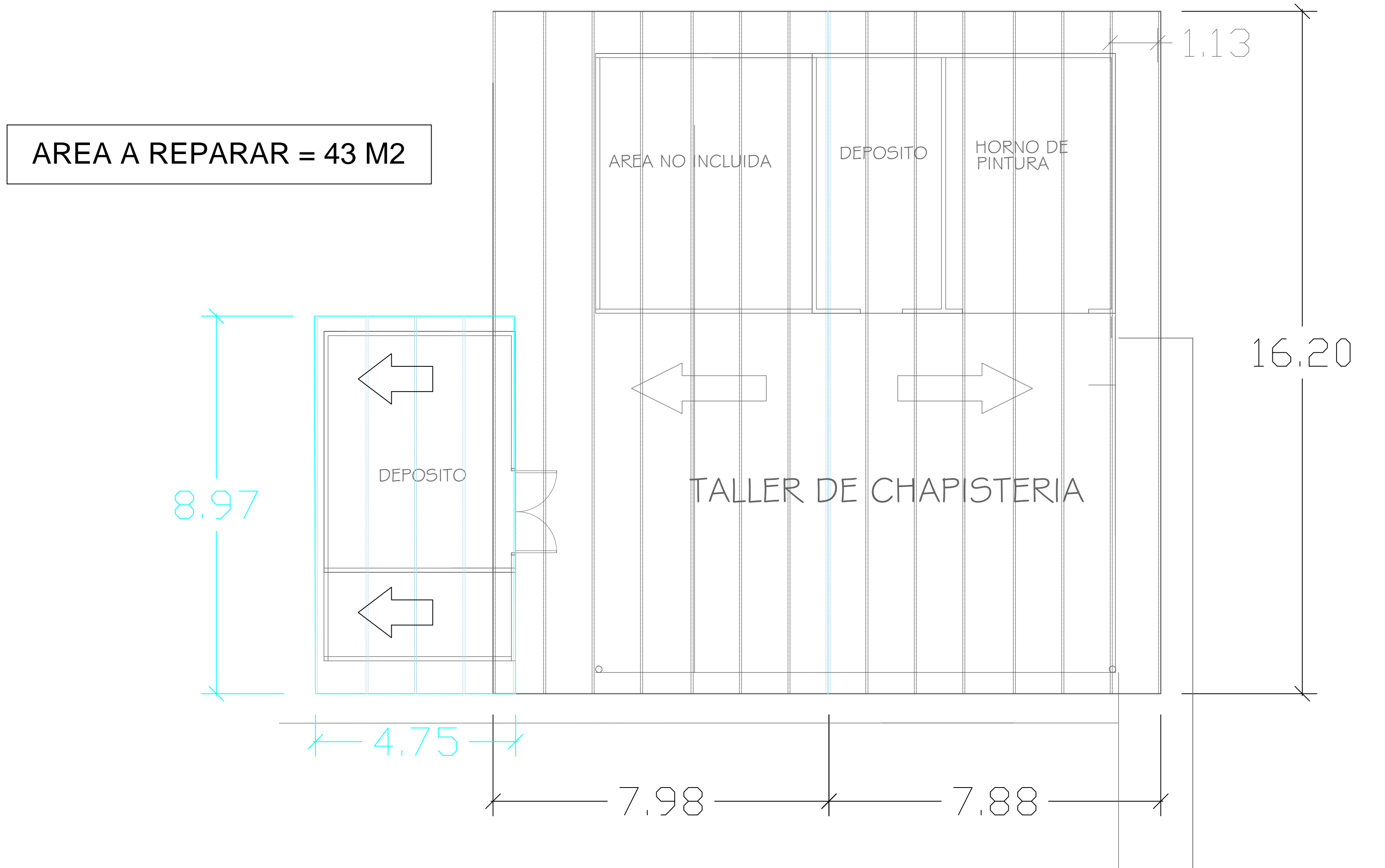
PLANTA DE TECHO (SIN ESCALA)
