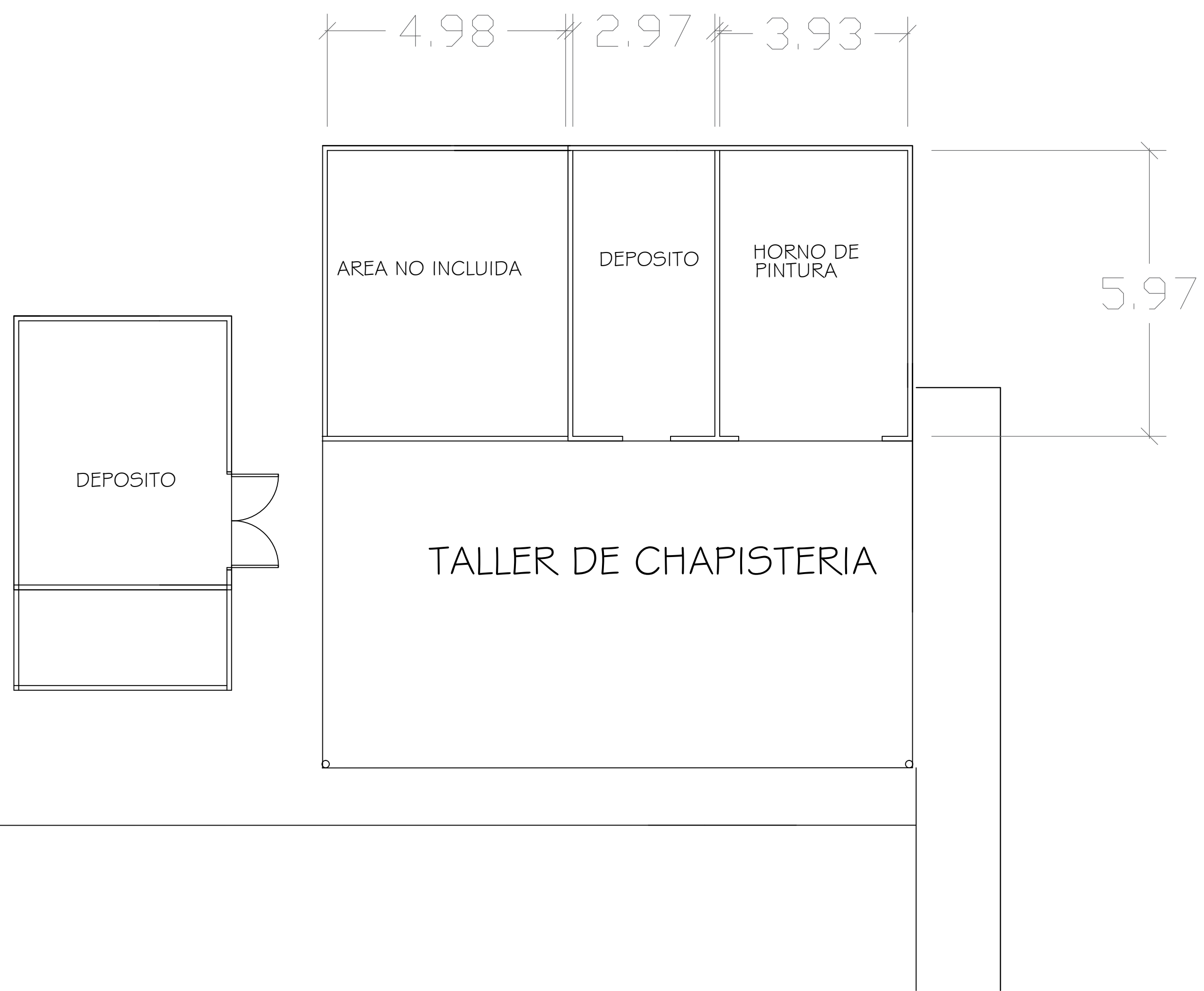
PLANTA ARQUITECTONICA (SIN ESCALA)
