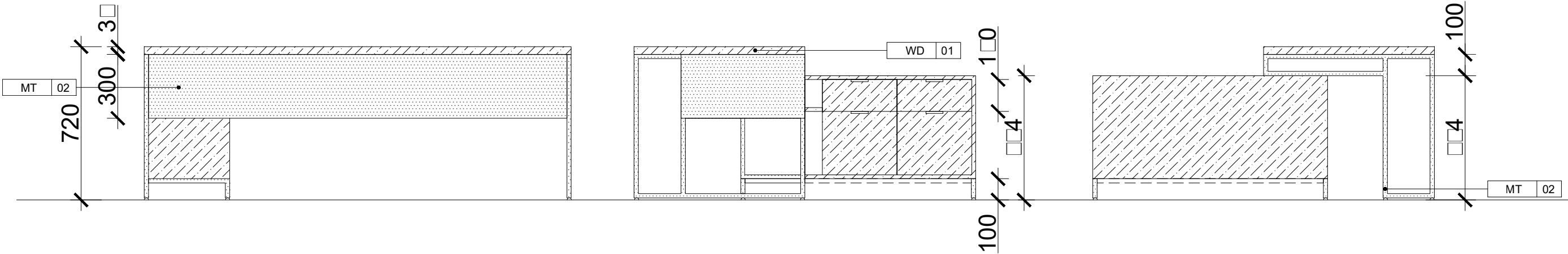
2 O T E 1 UN RC YEREVAN OFFICE SCALE 1:20
