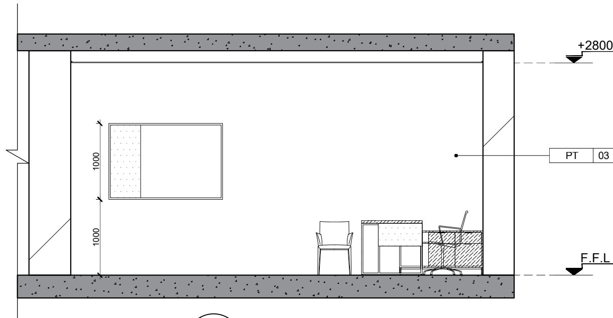
2 ELEVATION 4-a UN RC OFFICE YEREVAN SCALE 1:50
