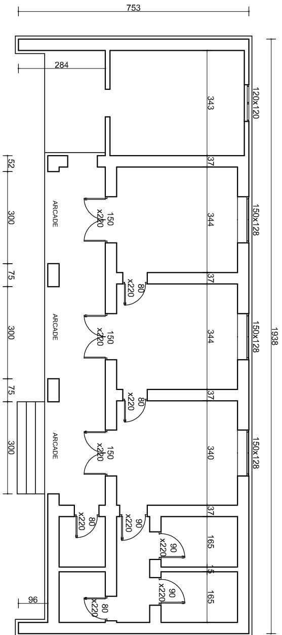
VUE EN PLAN BRIGADE TERRITORIALE DE BANGASSOU
