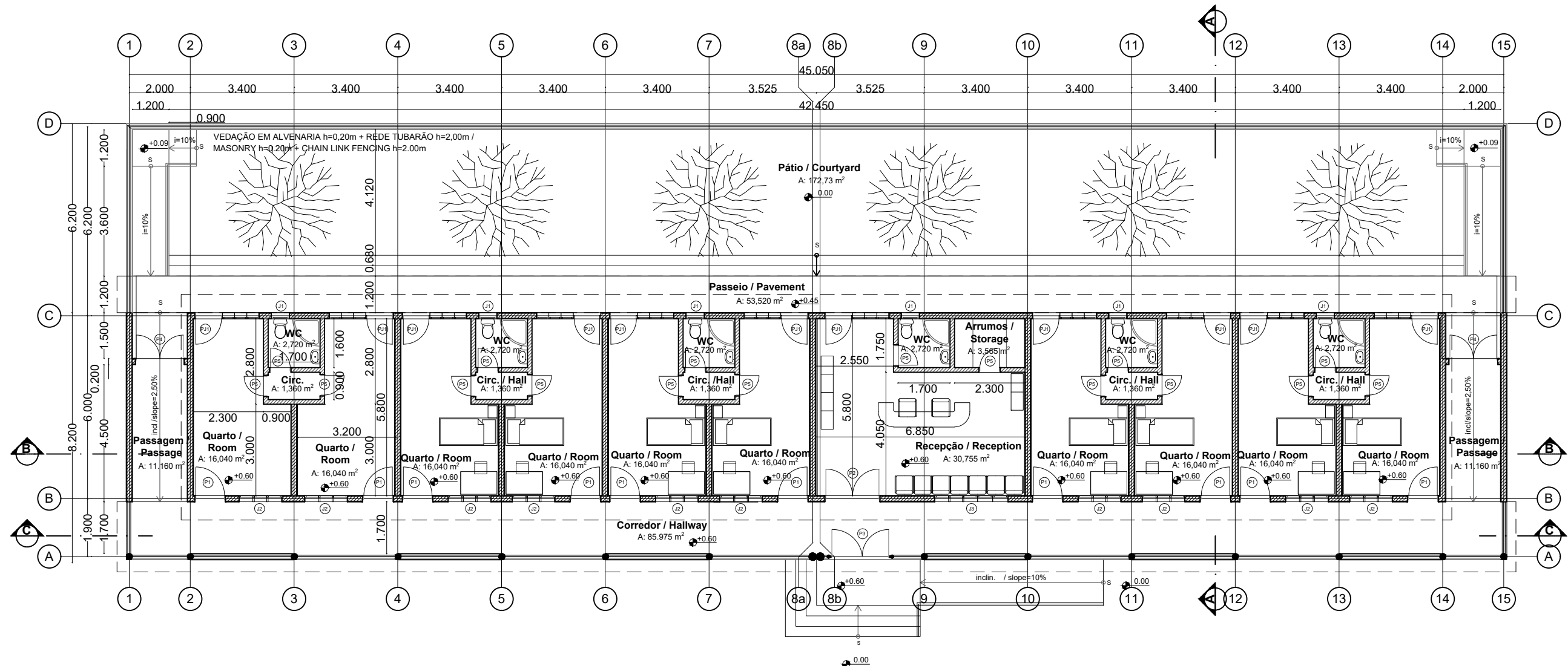
PLANTA DE PISO / FLOOR PLAN
