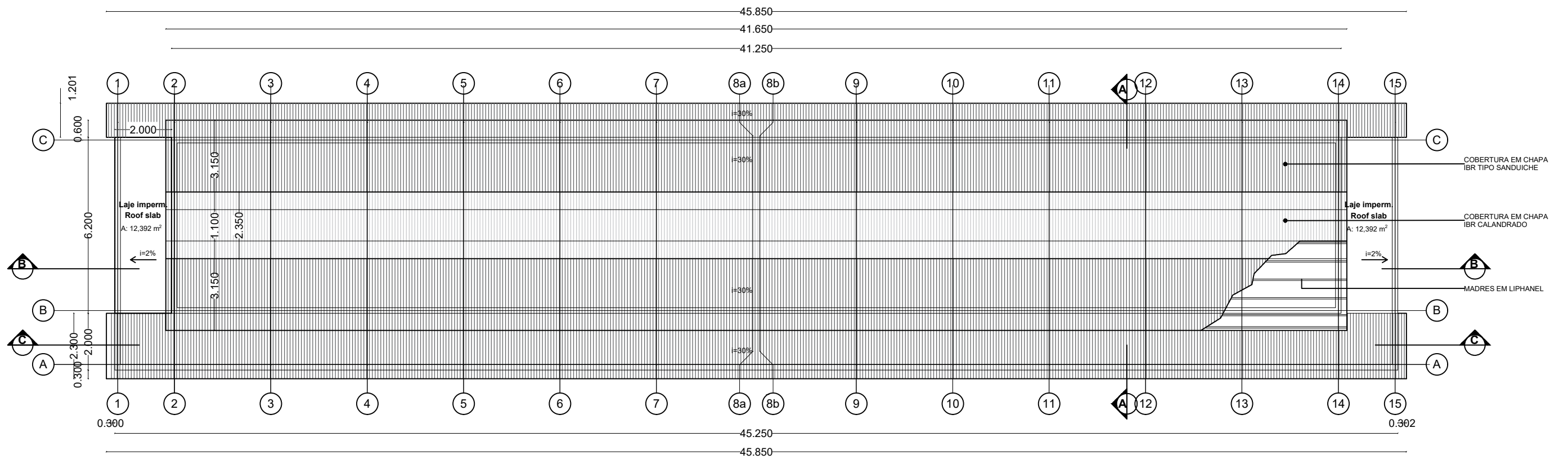
PLANTA DA COBERTURA / ROOF PLAN
