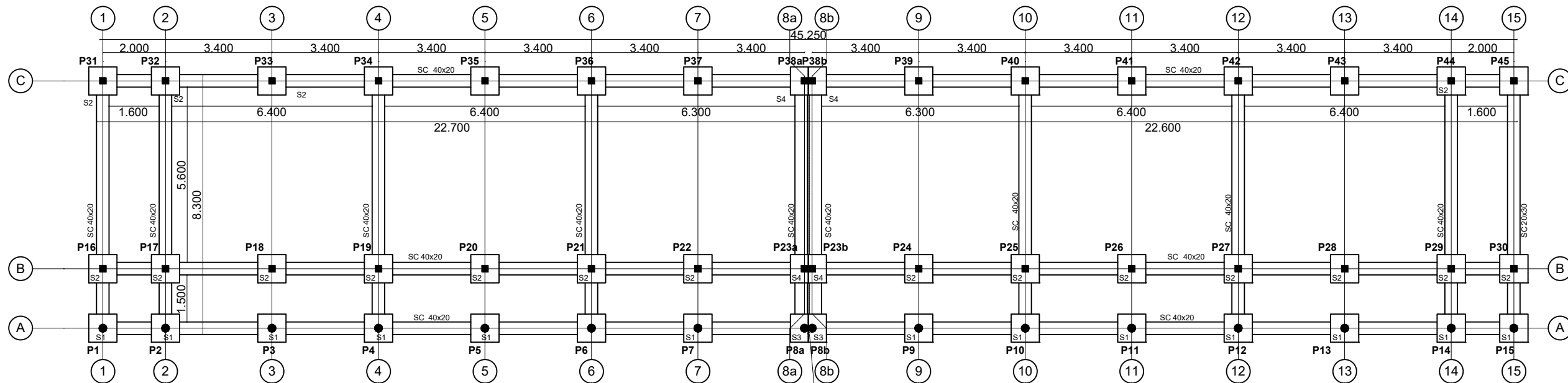
PLANTA DE FUNDAÇÃO / FOUNDATION LAYOUT
