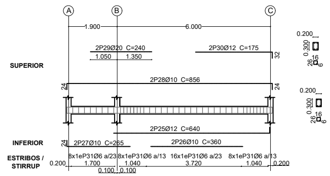
VIGA / BEAM V2
