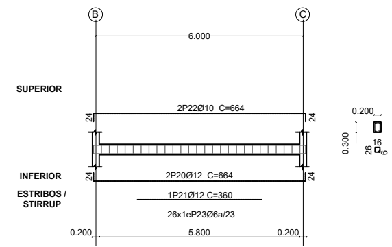
VIGA / BEAM V3
