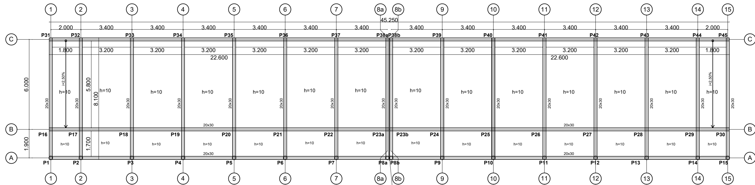
PLANTA ESTRUTURAL DA LAJE DE PAVIMENTO / GROUND FLOOR PLAN
