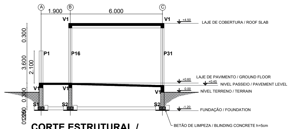
CORTE ESTRUTURAL / STRUCTURAL SECTION ESCALA / SCALE 1:150
