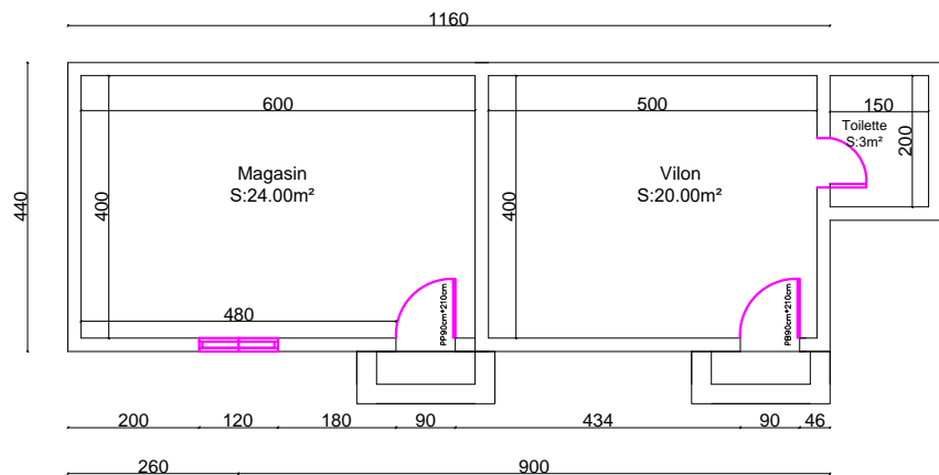
PLAN DE MACONNERIE
