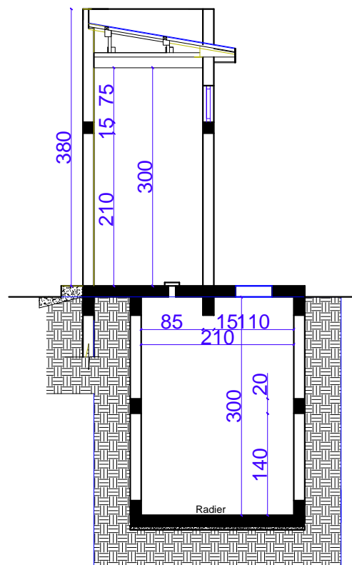
Coupe Transversale
