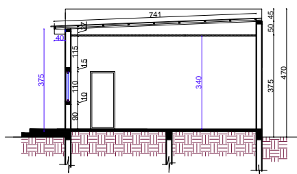
COUPE TRANSVERSALE
