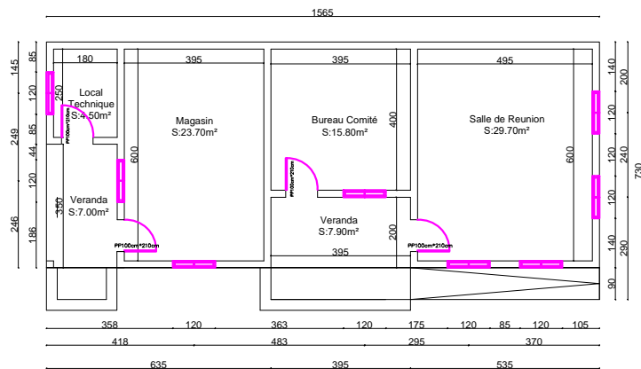
PLAN DE MAÇONNERIE
