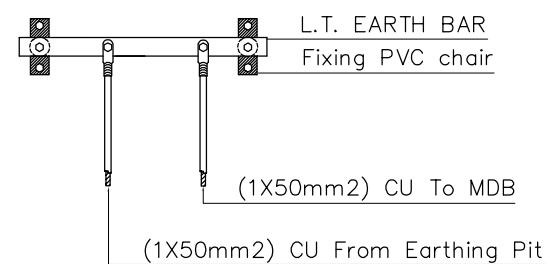
L.T. Earthing Bar
