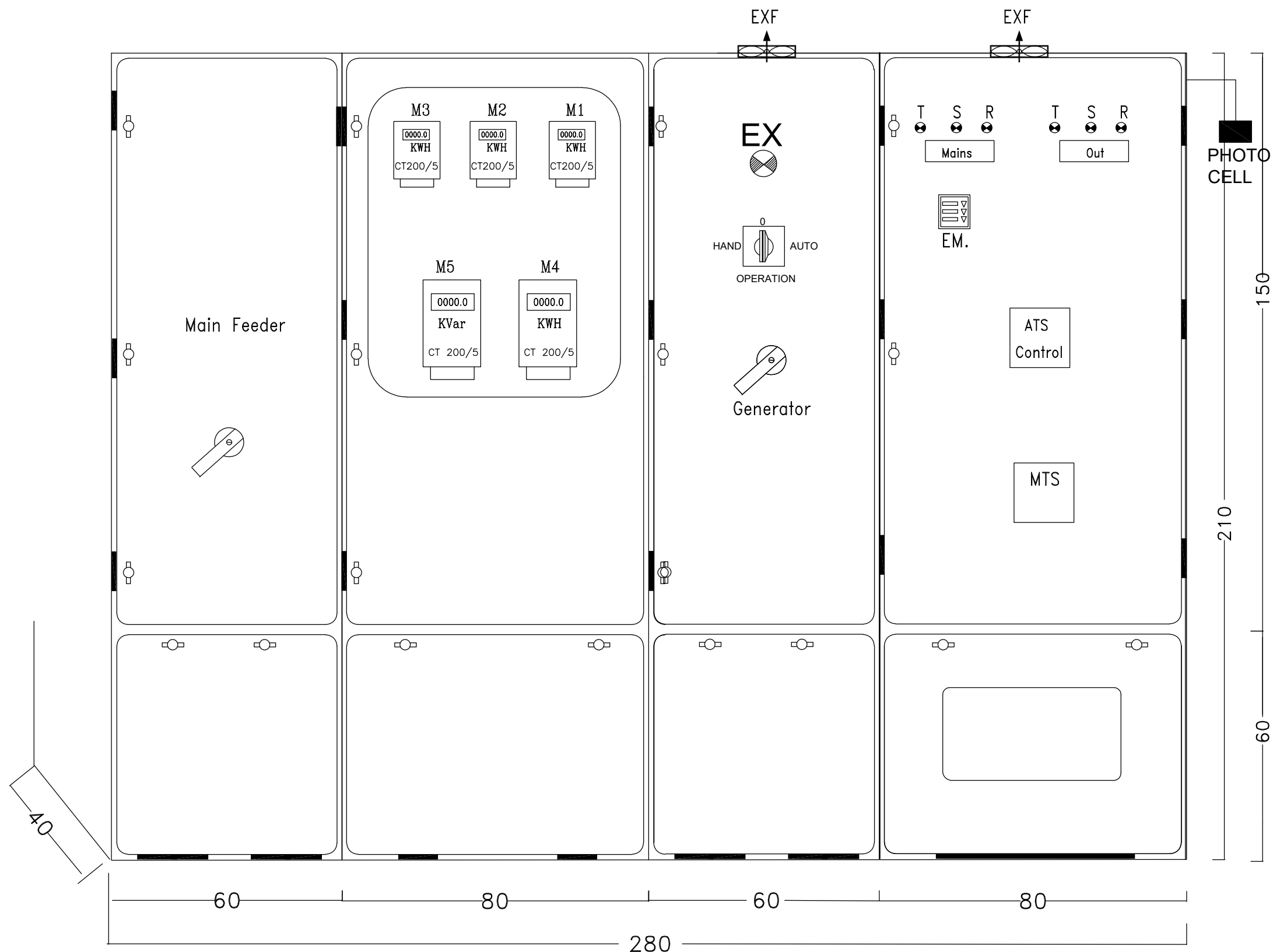
MDB LAYOUT
