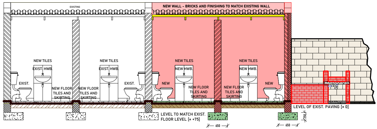
SECTION D-D
