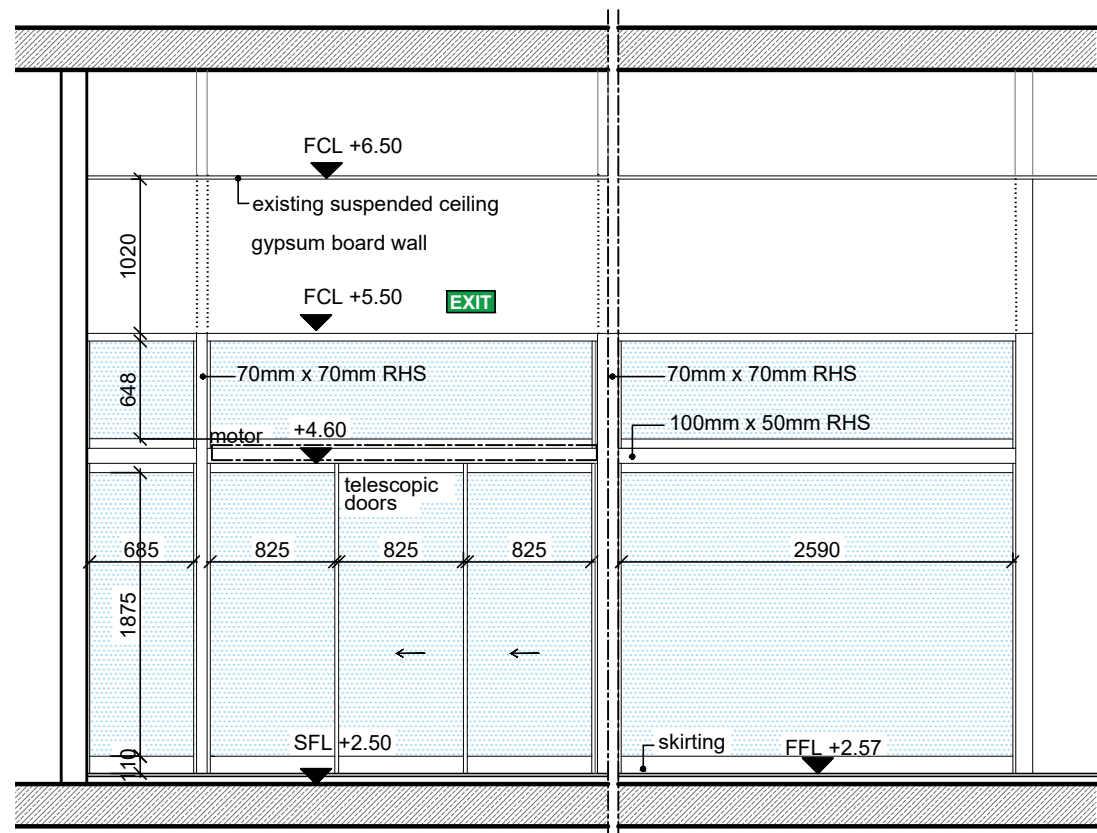
Section 1 1 : 50
