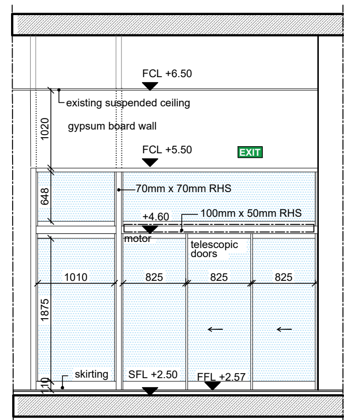
Section 2 1 : 50
