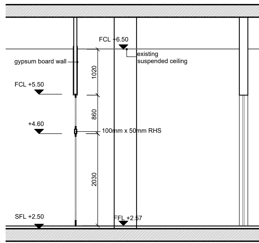
Section 4 1 : 50
