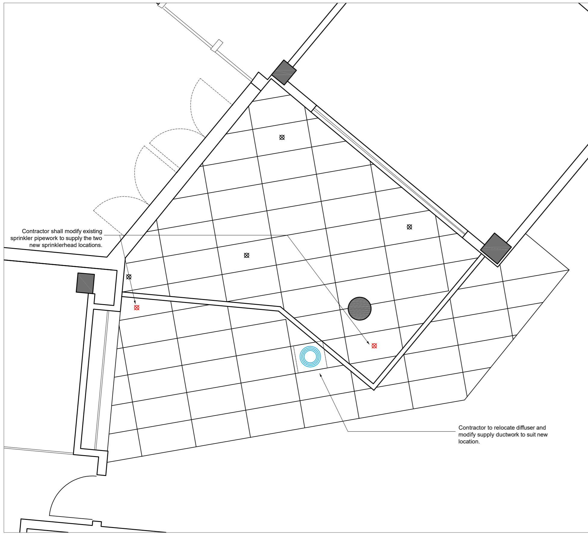
Ceiling Plan 1 : 50
