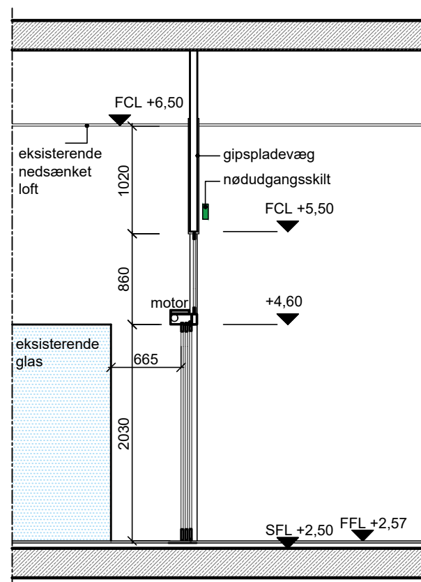
Sektion 3 1 : 50
