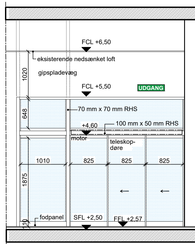
Sektion 2 1 : 50
