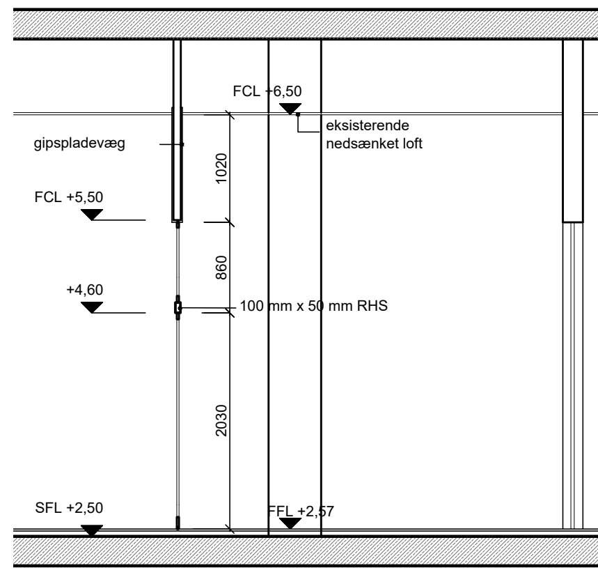
Sektion 4 1 : 50
