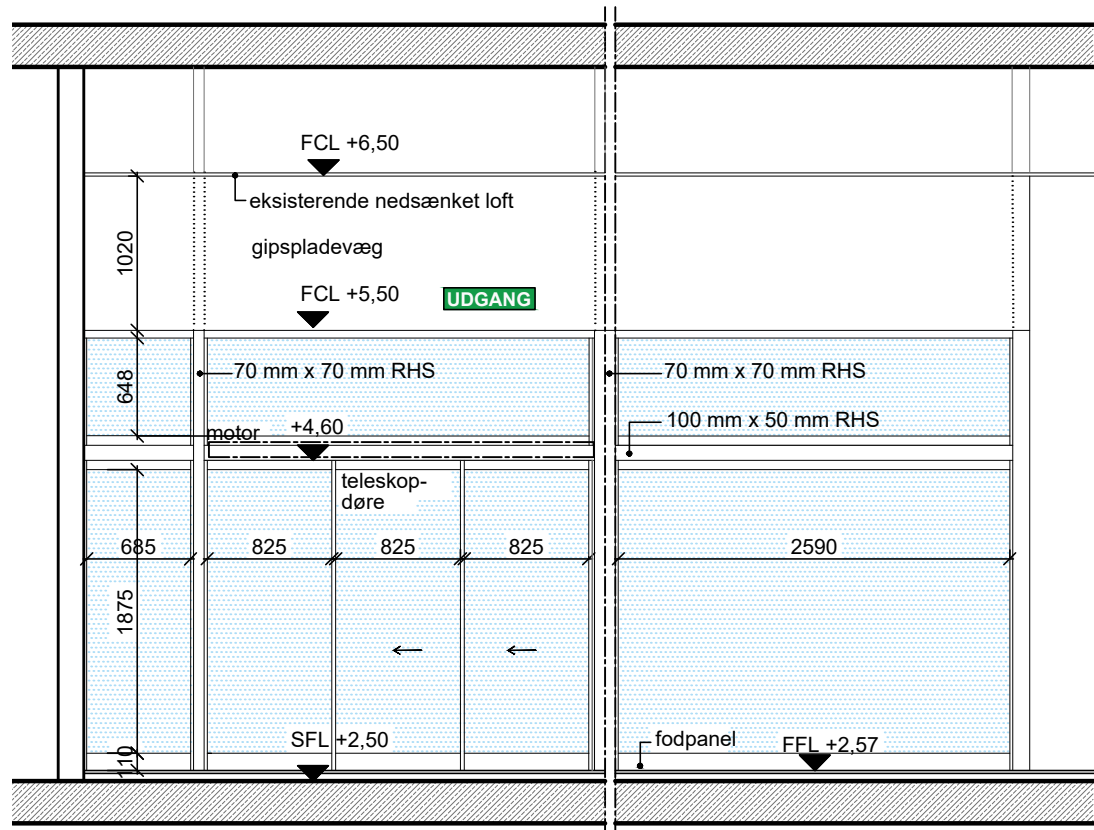
Sektion 1 1 : 50
