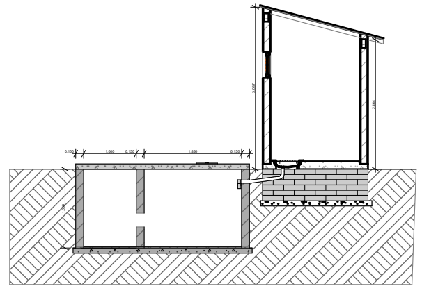
CORTE 1 1:100
