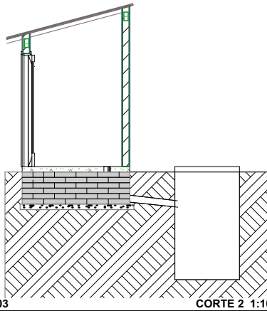
CORTE 2 1:100
