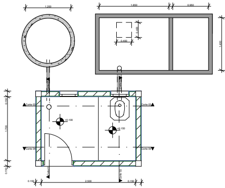
PLANTA BAIXA 1:100
